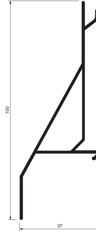
050001 LAMA Z / PVC SLAT Z / PVC LAME Z / PVC Escala 1:1 Scale 1:1 Echelle 1:1
