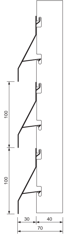
Instalación PC Installation PC 100 mm Installation PC
